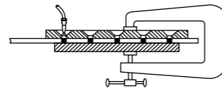
Lochplatte zum Richten von Dünnblechteilen
